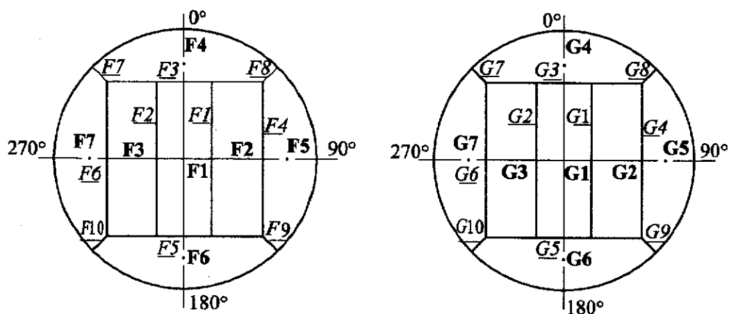
图 1 上、下极带板的编号和焊缝的编号
